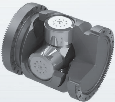
■ Yoke
