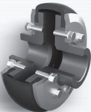
■ Rubber Coupling
